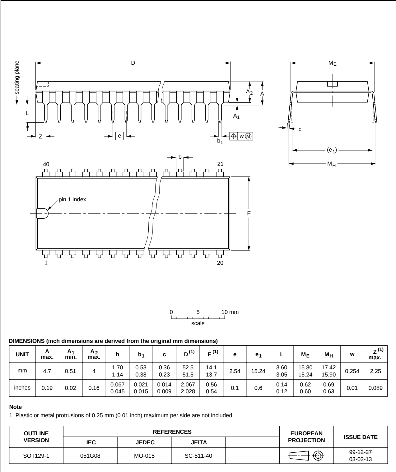
Fig 26. DIP40 (SOT129-1).
