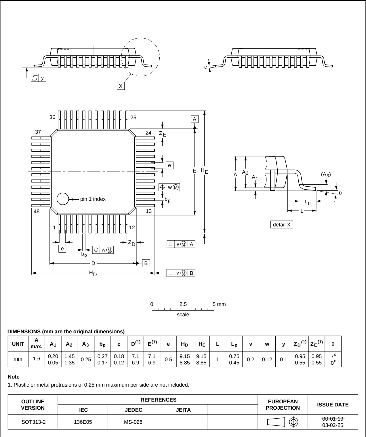
Fig 24. LQFP48 (SOT313-2).
